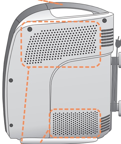
本体側面
